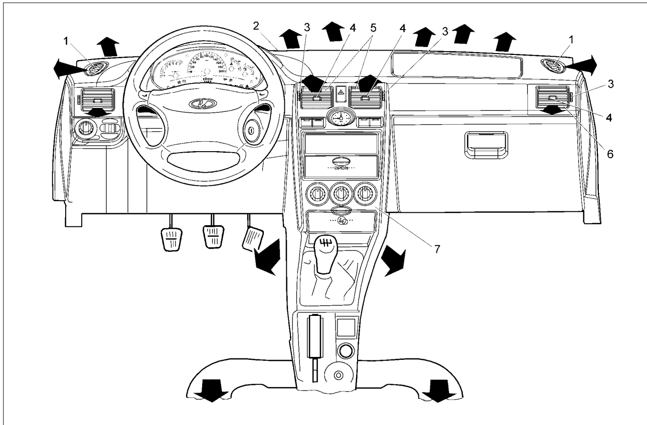
Рис. 38. Органы управления системой вентиляции и отопления салона
