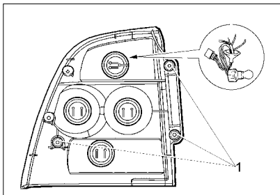
Рис. 55. Задний фонарь
