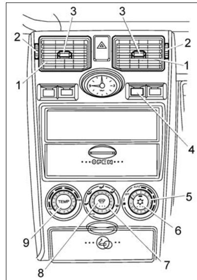
Рис. 39а. Органы управления
