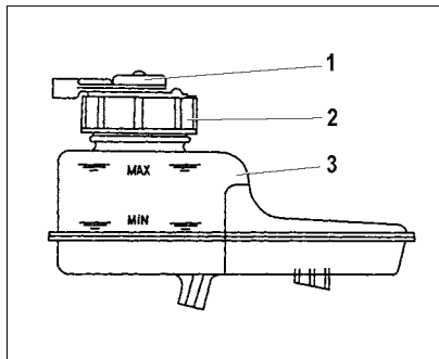
Рис. 45. Бачок гидропровода тормозов
