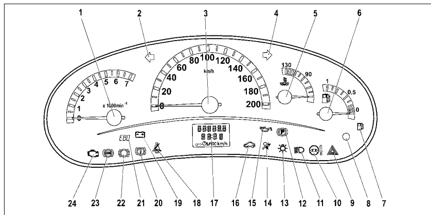
Рис. 31. Комбинация приборов
