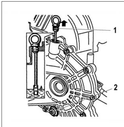
Рис. 43. Проверка уровня масла в коробке передач
