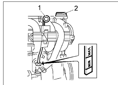
Рис. 42. Проверка уровня масла в картере двигателя
