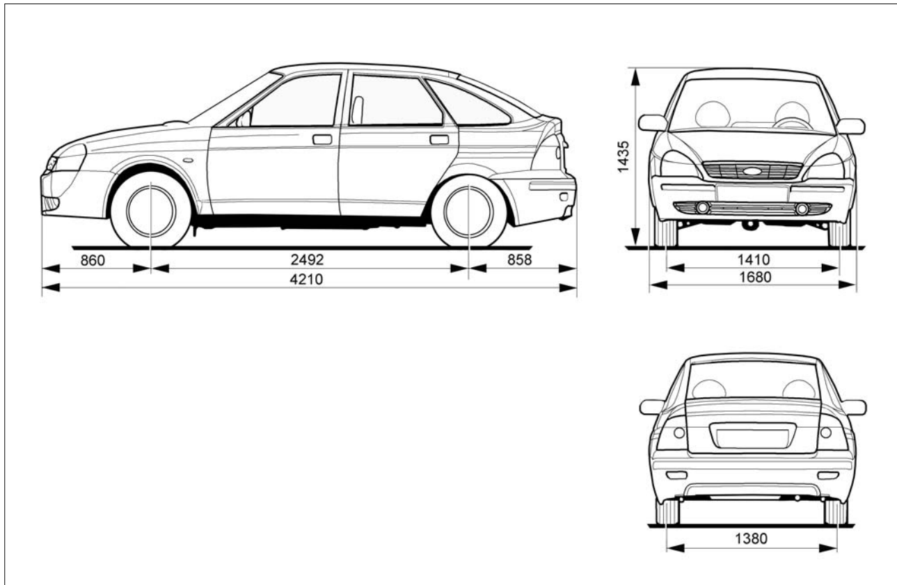
Рис. 62. Габаритные размеры (справочные) автомобиля LADA PRIORA хэтчбек
