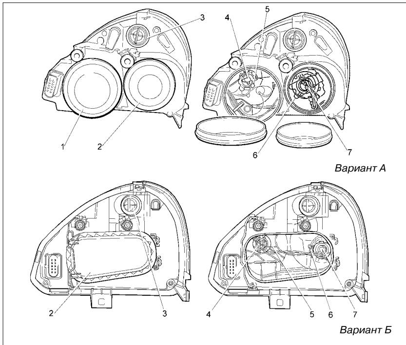
Рис. 54. Блок-фара
