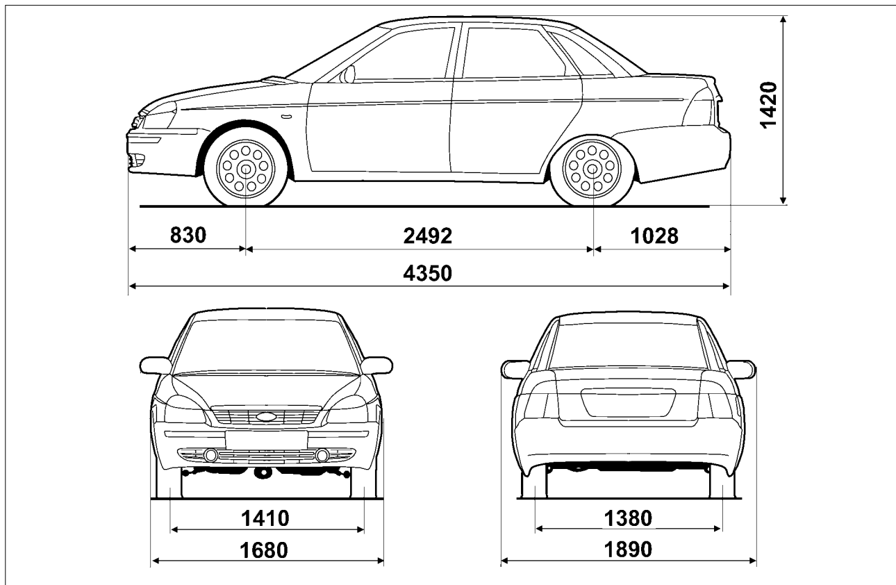
Рис. 61. Габаритные размеры (справочные) автомобиля LADA PRIORA и его модификаций
