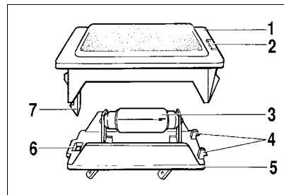
Рис. 60. Плафон освещения вещевого ящика
