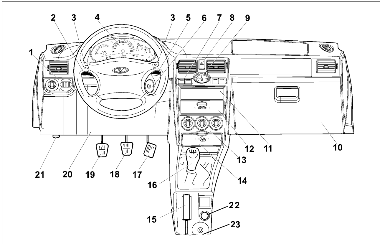
Рис. 30. Органы управления и приборы
