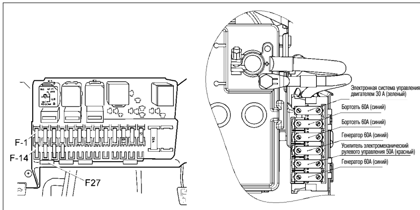
Рис. 53. Монтажный блок и блок предохранителей в моторном отсеке
