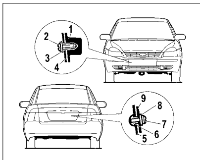
Рис. 40. Установка номерных знаков
